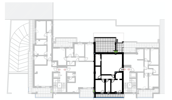
Piano Terzo
